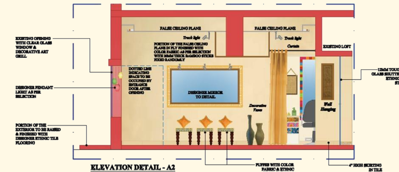
dd : ELEVATION DETAIL – BOUTIQUE
