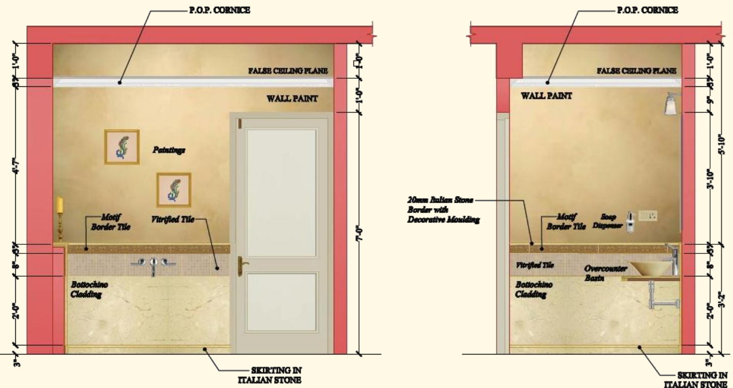
dd : ELEVATION DETAIL
