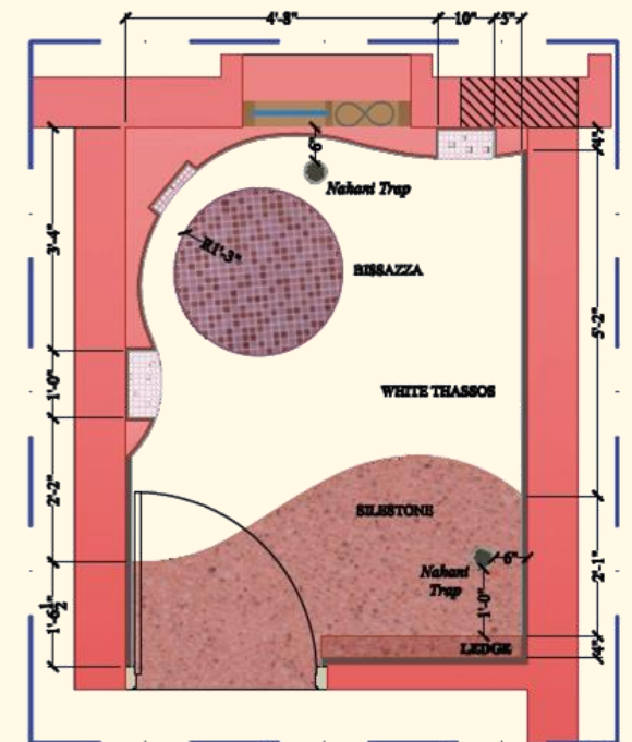
dd : FLOORING PLAN
