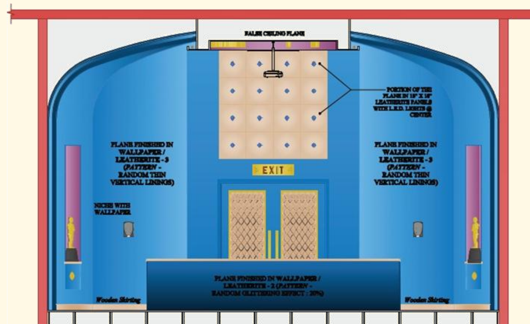
dd : ELEVATION DETAIL
