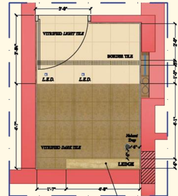
dd : FLOORING PLAN
