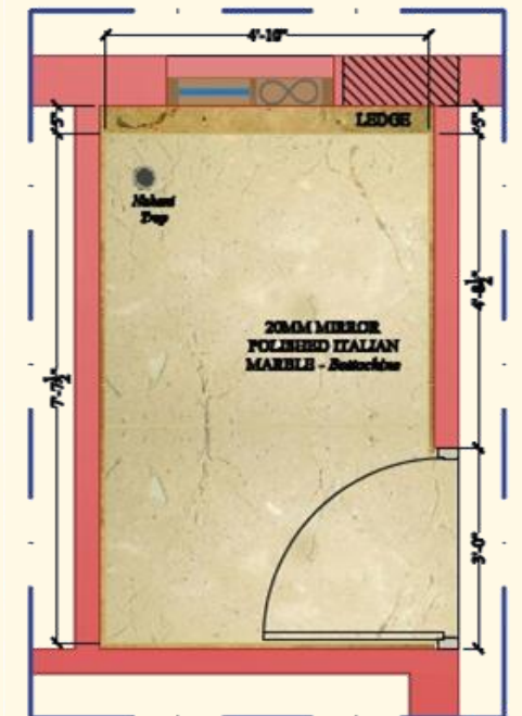
dd : FLOORING PLAN
