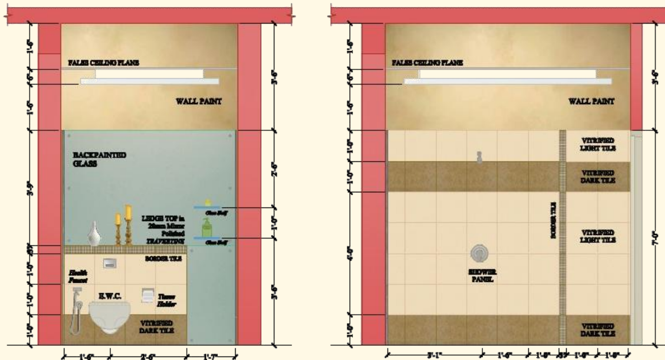
dd : ELEVATION DETAIL
