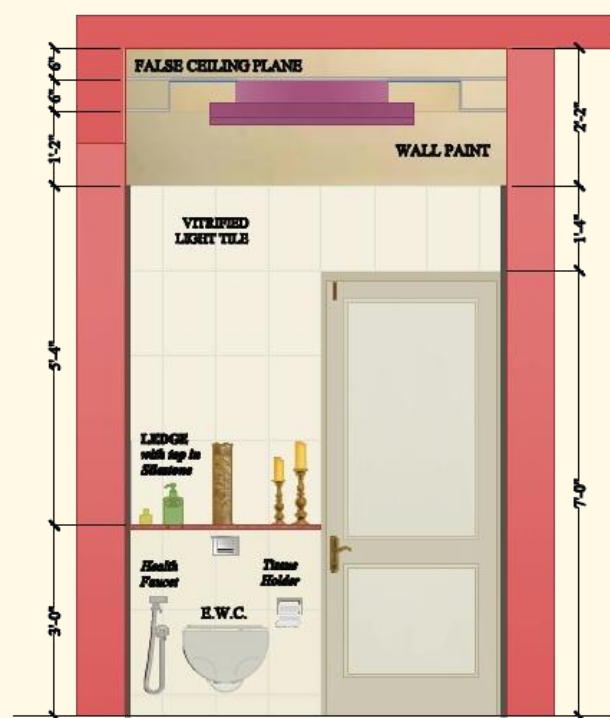
dd : ELEVATION DETAIL
