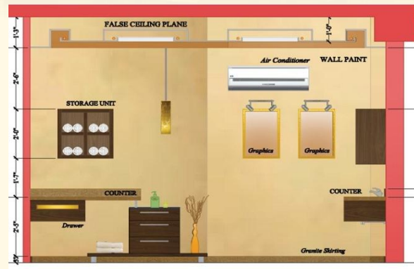
dd : ELEVATION DETAIL – SPA 1
