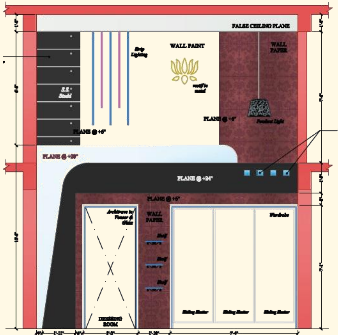
dd : SON'S BEDROOM - DOUBLE HEIGHT WALL
