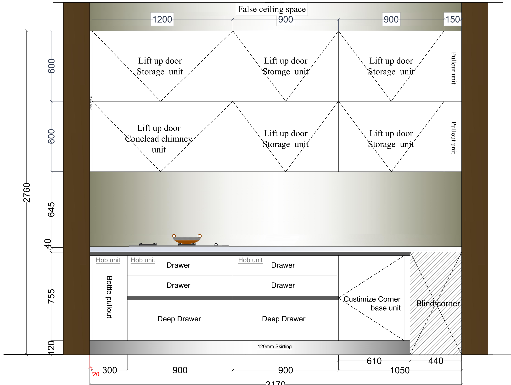
Elevation : A
