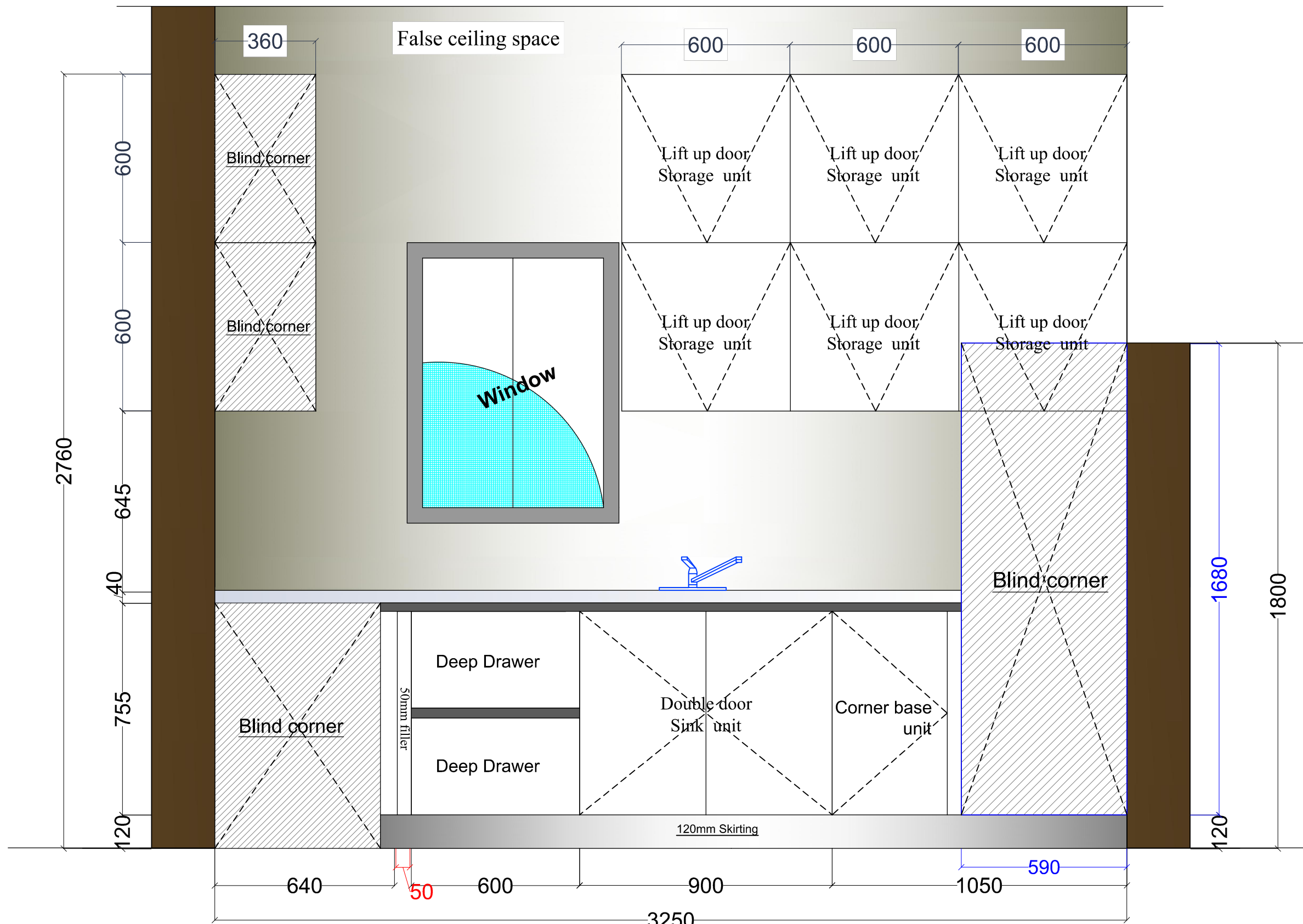
Elevation : B
