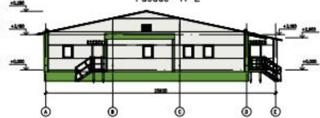
Facade A-E
