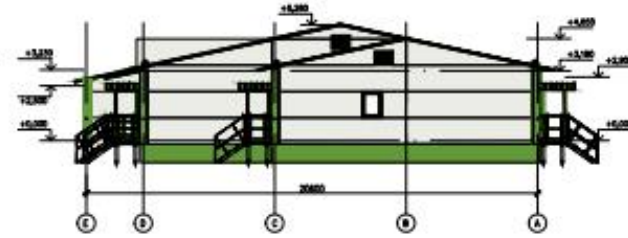
Facade E-A
